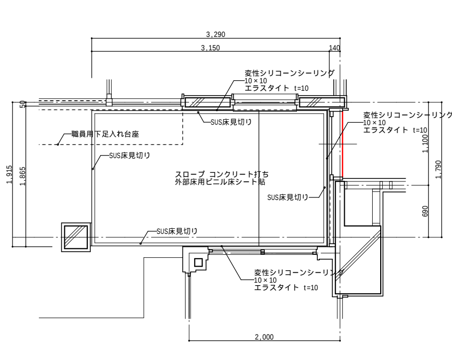
スロープ平面図 S=1:50
