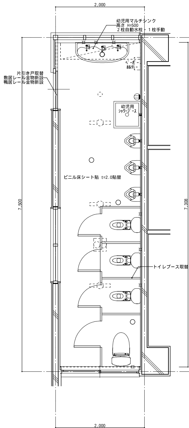
2階 幼児用便所 平面図
