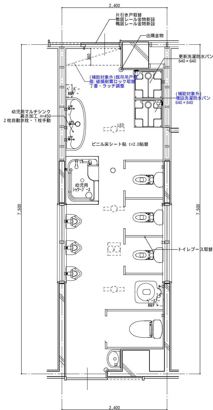
1階 幼児用便所 平面図
