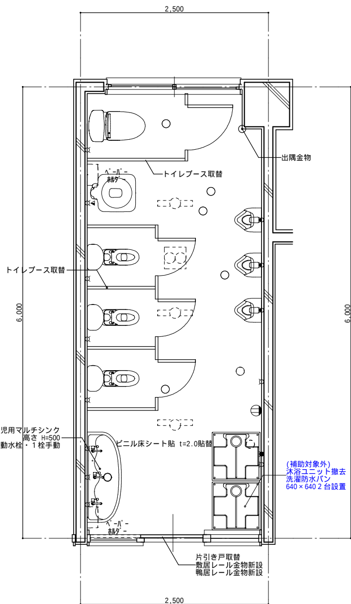
2階 幼児用便所 平面図
