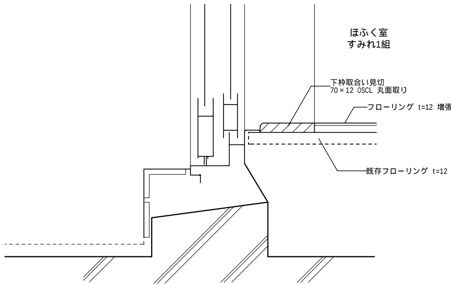
アルミ下枠取合い見切詳細図 S=1:5
