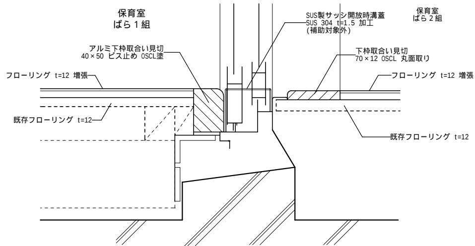
アルミ下枠取合い見切詳細図 S=1:5
