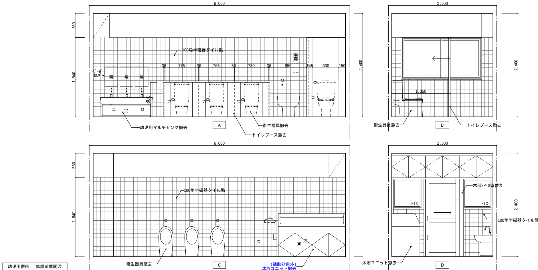
幼児用便所 修繕前展開図
