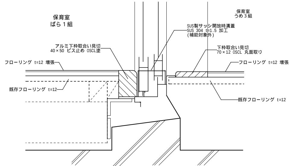
アルミ下枠取合い見切詳細図 S=1:5
