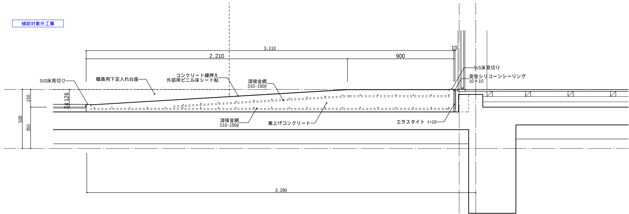
スロープ断面詳細図 S=1:20
